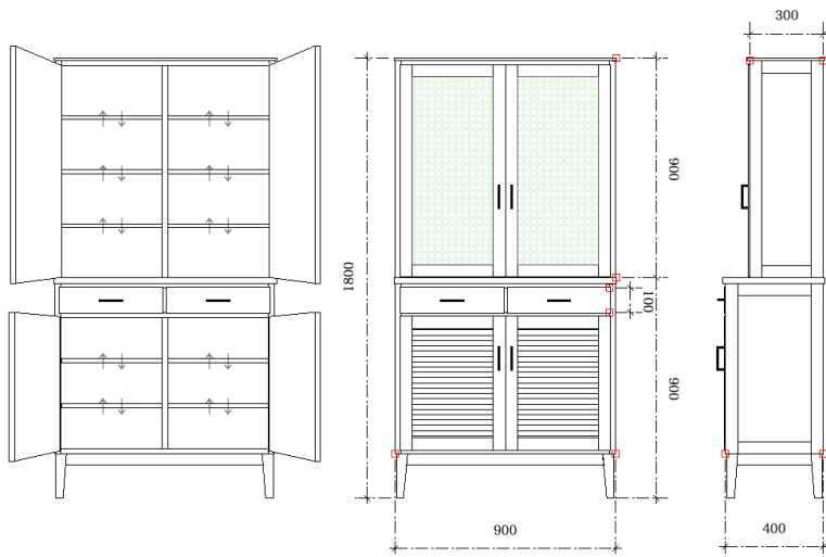
画像商品図面 w900 d400(上段300) h1800 / 上段型ガラス・下段ガラリ扉・脚仕様
